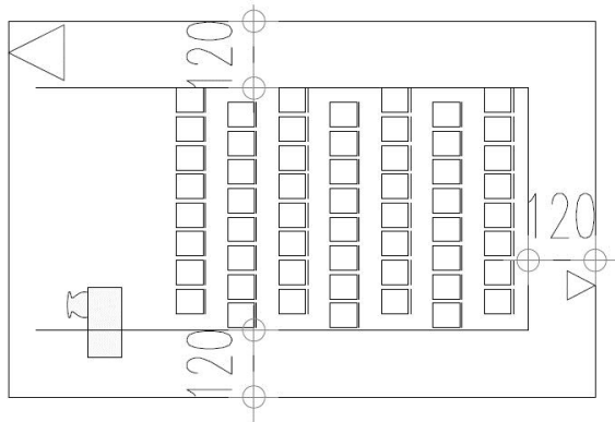
VARIANTE THEATER SEMINARRAUM 1 56 Personen
